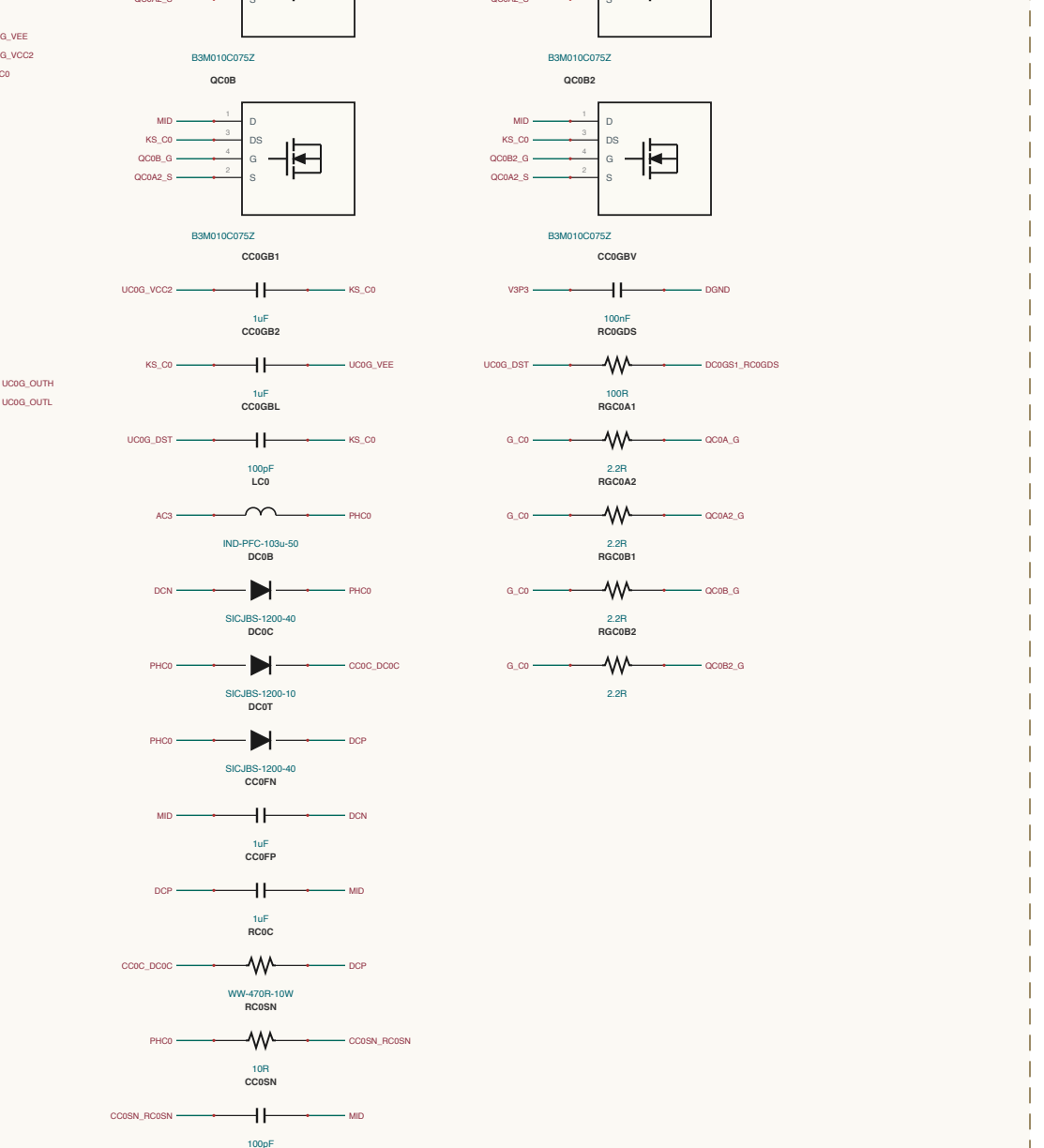
DC-LINK / LINK-BANK-0
